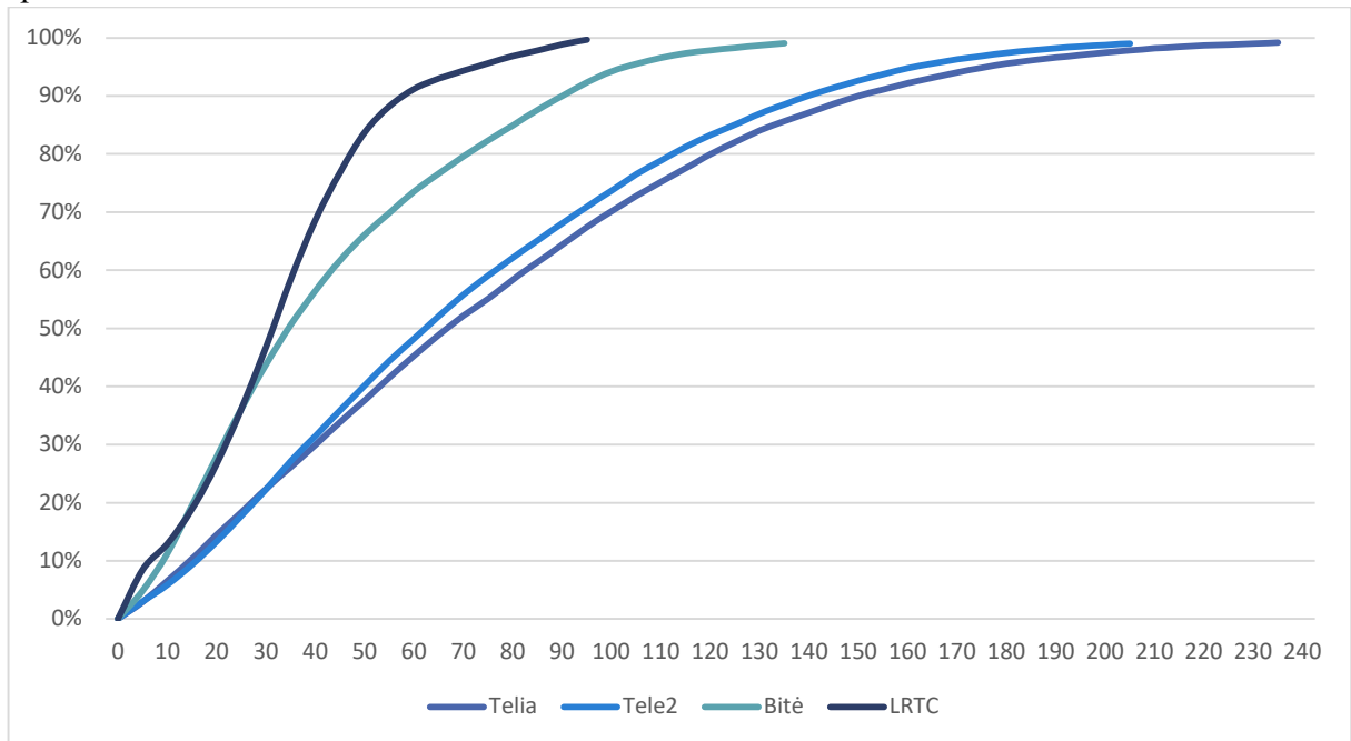
3 pav. Duomenų gavimo spartos miestuose ir keliuose verčių suminis procentinis pasiskirstymas, Mb/s
