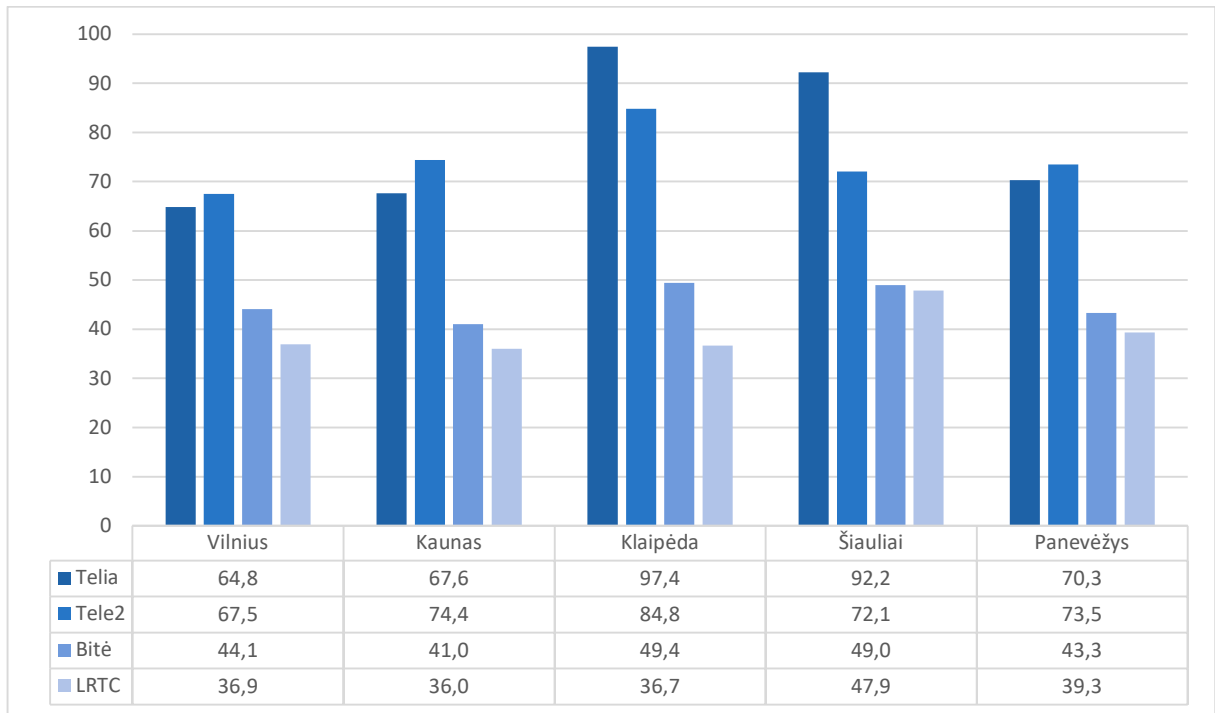
10 pav. Duomenų gavimo spartos vidutinių verčių palyginimas didžiuosiuose miestuose, Mb/s
