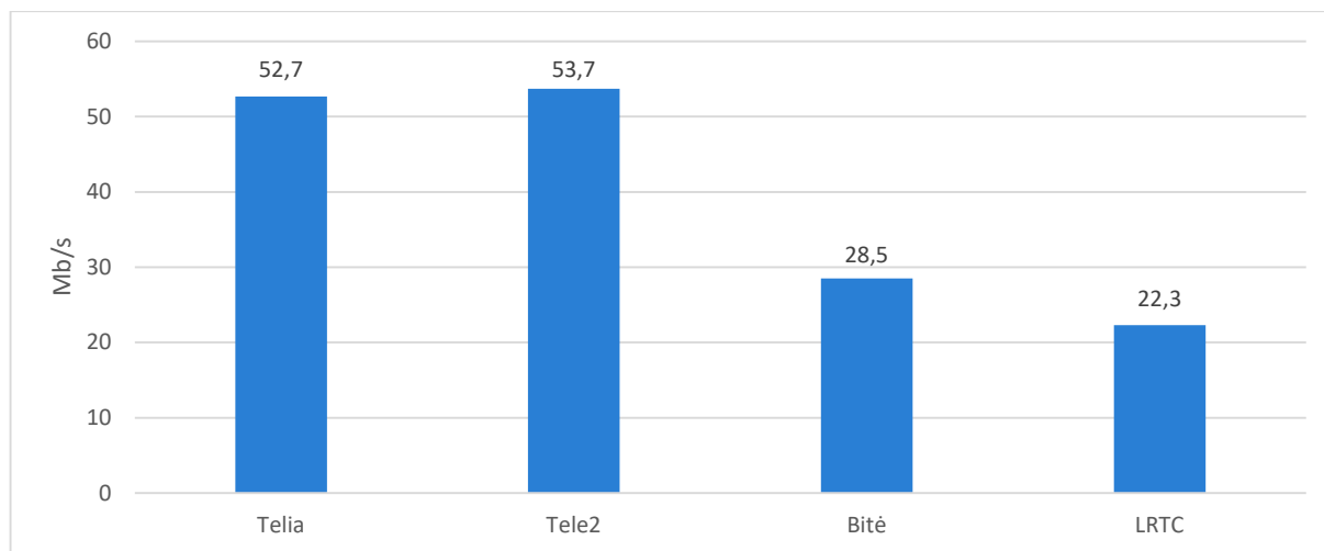
5 pav. Vidutinė duomenų gavimo sparta matuojant geležinkelių keleiviniuose maršrutuose, Mb/s
